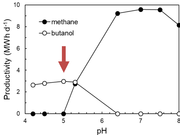
Butanol Productivity
